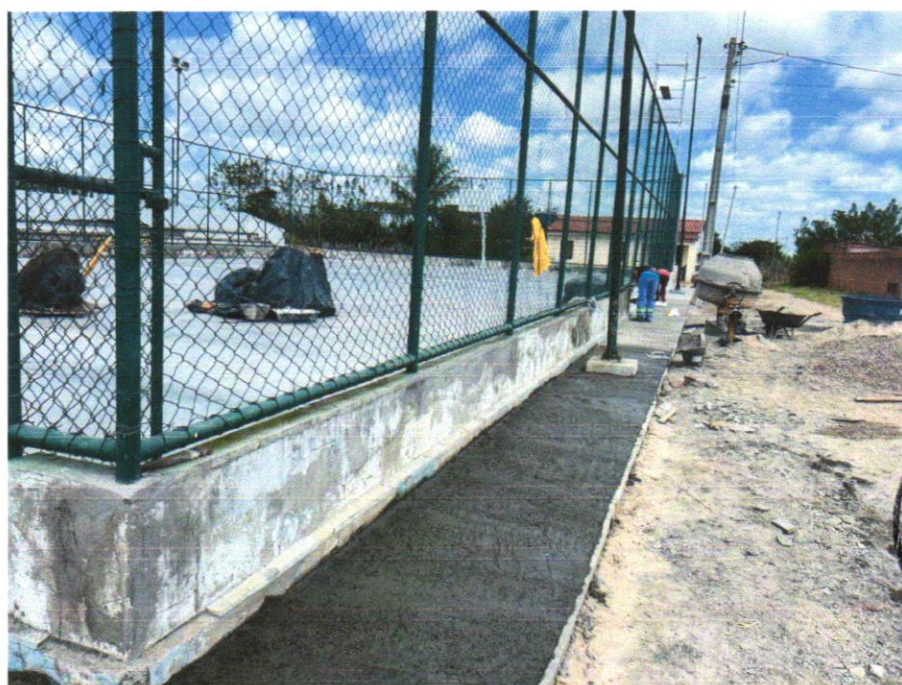
Foto 10 - ALAMBRADO PARA QUADRA POLIESPORTIVA, ESTRUTURADO POR TUBOS DE AÇO GALVANIZADO, (MONTANTES COM DIÂMETRO 2", TRAVESSAS E ESCORAS COM DIÂMETRO 1 ¼ ), COM TELA DE ARAME GALVANIZADO, FIO 10 BWG E MALHA QUADRADA 5X5CM (EXCETO MURETA). AF_03/2021
